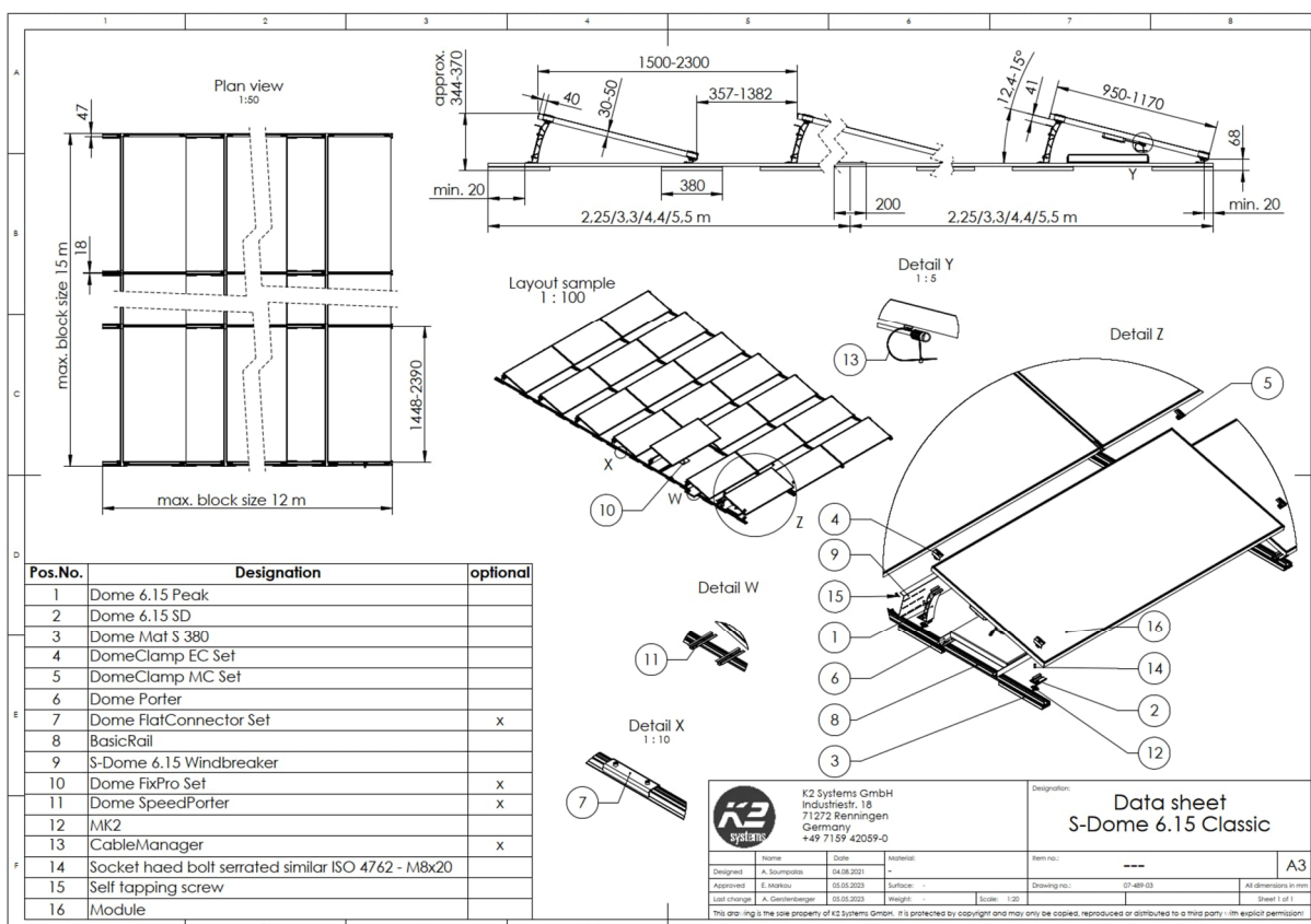
Bild 5: Systemdatenblatt des PV-Flachdachsystems "S-Dome 6.15 Classic"
