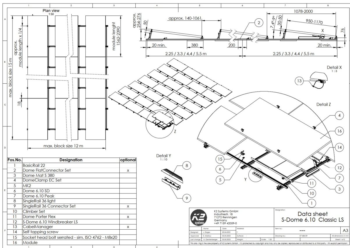
Bild 2: Systemdatenblatt des PV-Flachdachsystems "S-Dome 6.10 Classic LS"
