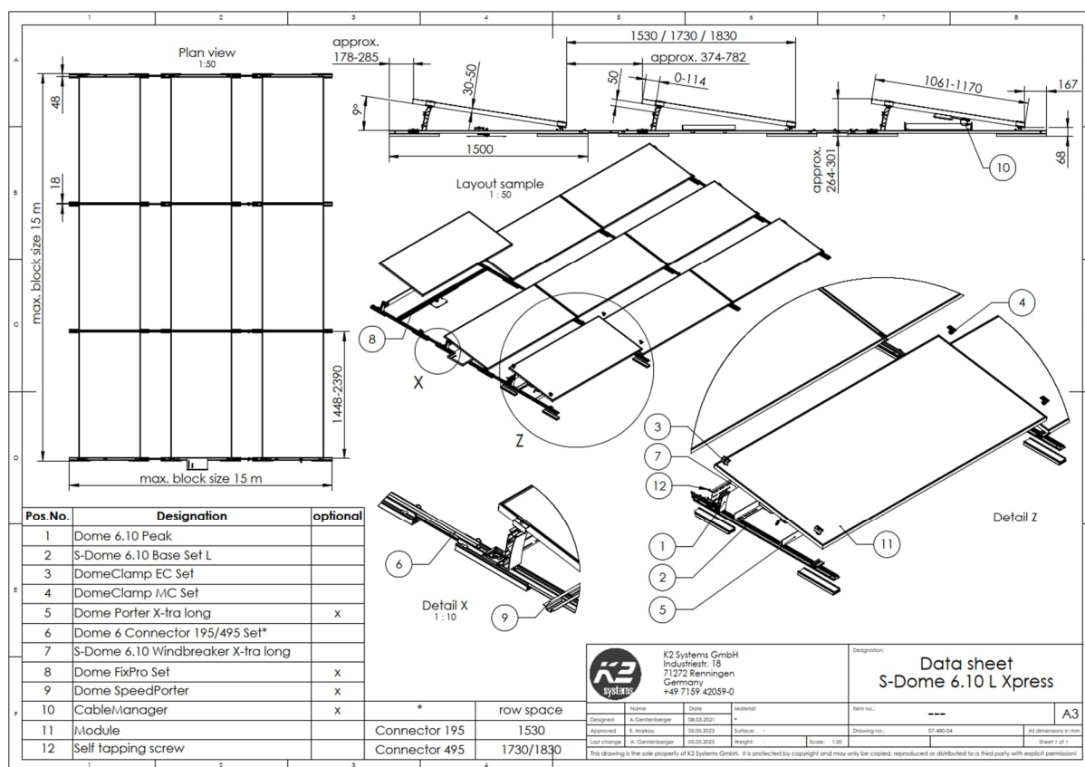
Bild 4: Systemdatenblatt des PV-Flachdachsystems "S-Dome 6.10 L Xpress"
