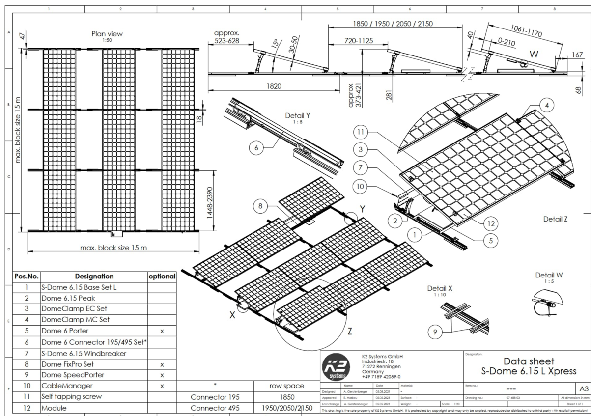
Bild 7: Systemdatenblatt des PV-Flachdachsystems "S-Dome 6.15 L Xpress"
