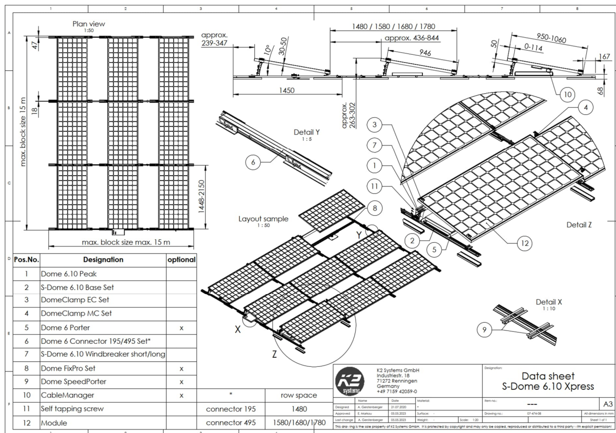
Bild 3: Systemdatenblatt des PV-Flachdachsystems "S-Dome 6.10 Classic Xpress"
