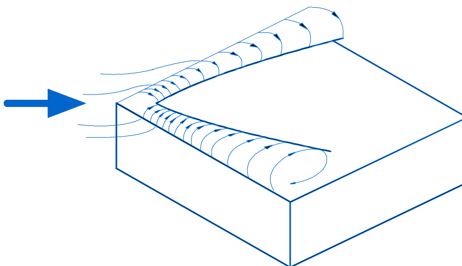
Bild 8: Wirbel, die durch Schräganströmung von der windzugewandten Dachecke ausgehen, führen zu Spitzensogwerten auf Flachdächern und darauf montierten Solarmodulen
