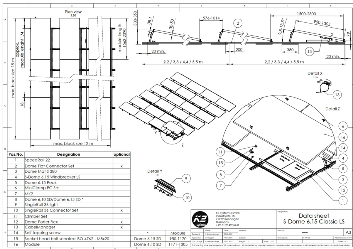
Bild 6: Systemdatenblatt des PV-Flachdachsystems "S-Dome 6.15 Classic LS"
