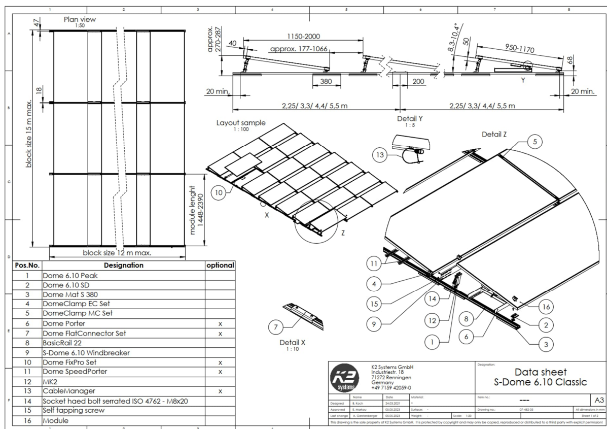
Bild 1: Systemdatenblatt des PV-Flachdachsystems "S-Dome 6.10 Classic"
